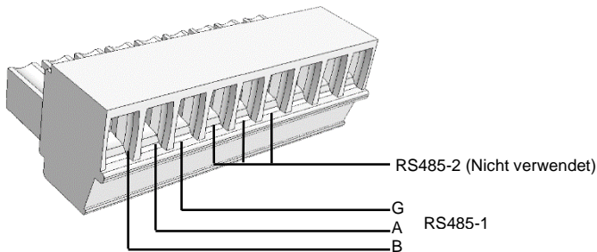
Abbildung 14: RS485-Klemmleiste
