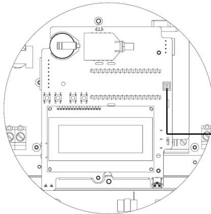
Abbildung 16: RS485-Terminierungsschalter
