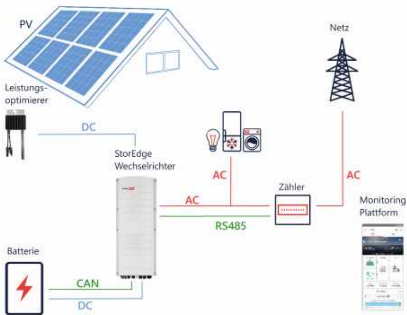
Abbildung 1: StorEdge Systemkomponenten
