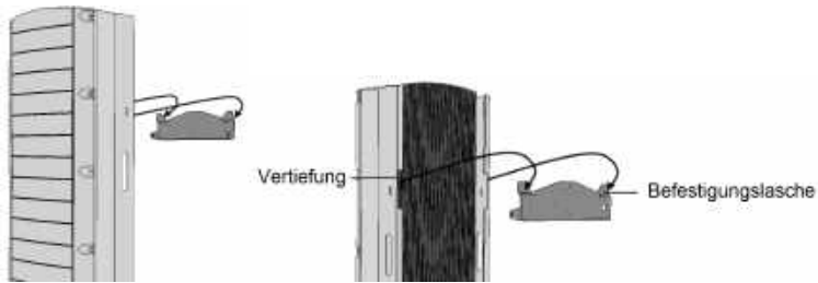
Abbildung 9: Aufhängen des Wechselrichters auf der Halterung
