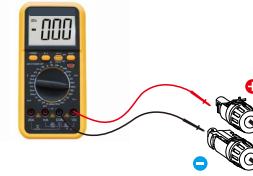
Abbildung 5.17 Multimetermessung
