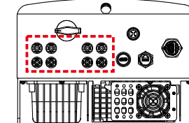
Abbildung 5.18 Verbindung des Gleichstromsteckers mit dem Wechselrichter
