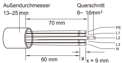
Abbildung 5.20 Abisolierter und entblößter Draht
