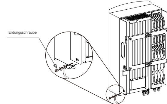
Abbildung 5.10 Befestigtes Kabel
