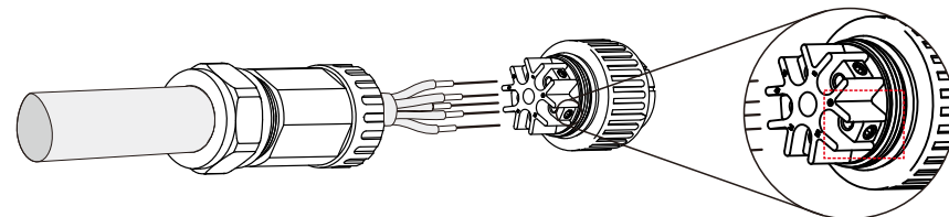
Abbildung 5.22 Angeschlossenes Kabel
