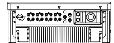
Abbildung 5.22 Verbindung des Gleichstromsteckers mit dem Wechselrichter
