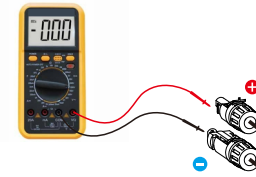
Abbildung 5.21 Multimetermessung
