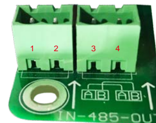
Abbildung 5.27 Belegung der RS485-Klemme
