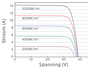
Stroom-spanningscurve JAM54D40-440/LB
