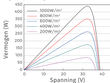
Vermogen-spanningscurve JAM54D40-440/LB
