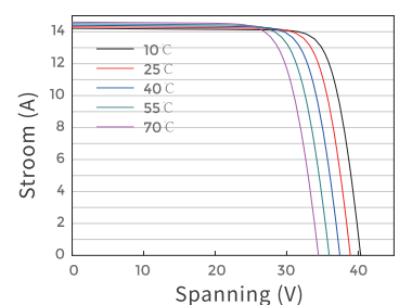
Stroom-spanningscurve JAM54D40-440/LB
